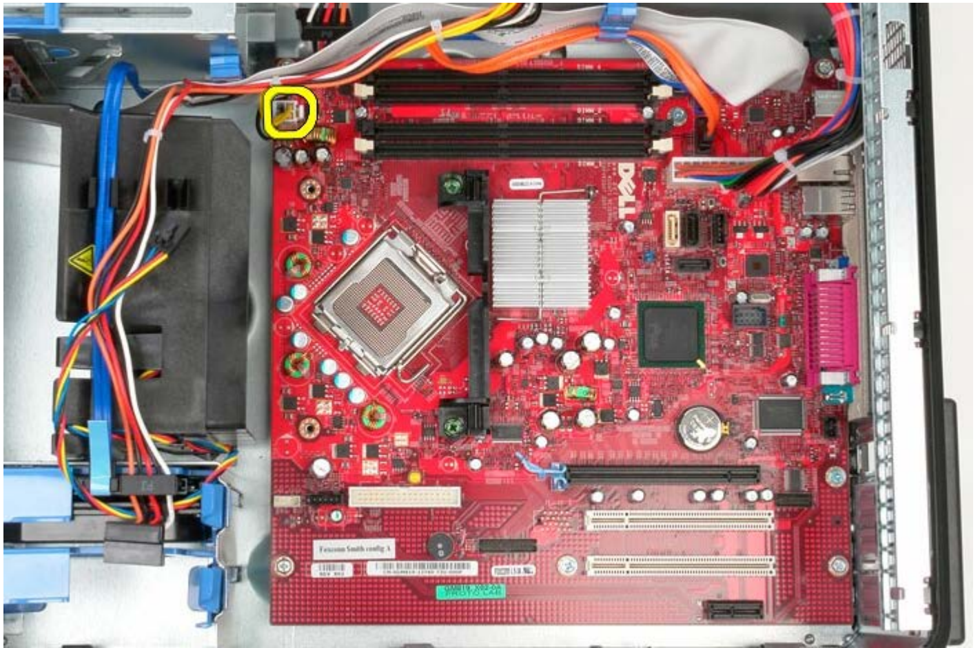
1 11 メインシステム基板の電源ケーブルを取り外します。
