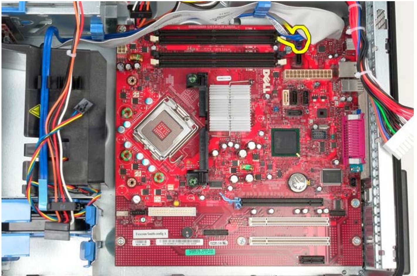
11 11 ハードドライブのデータケーブルを片付けておきます。
