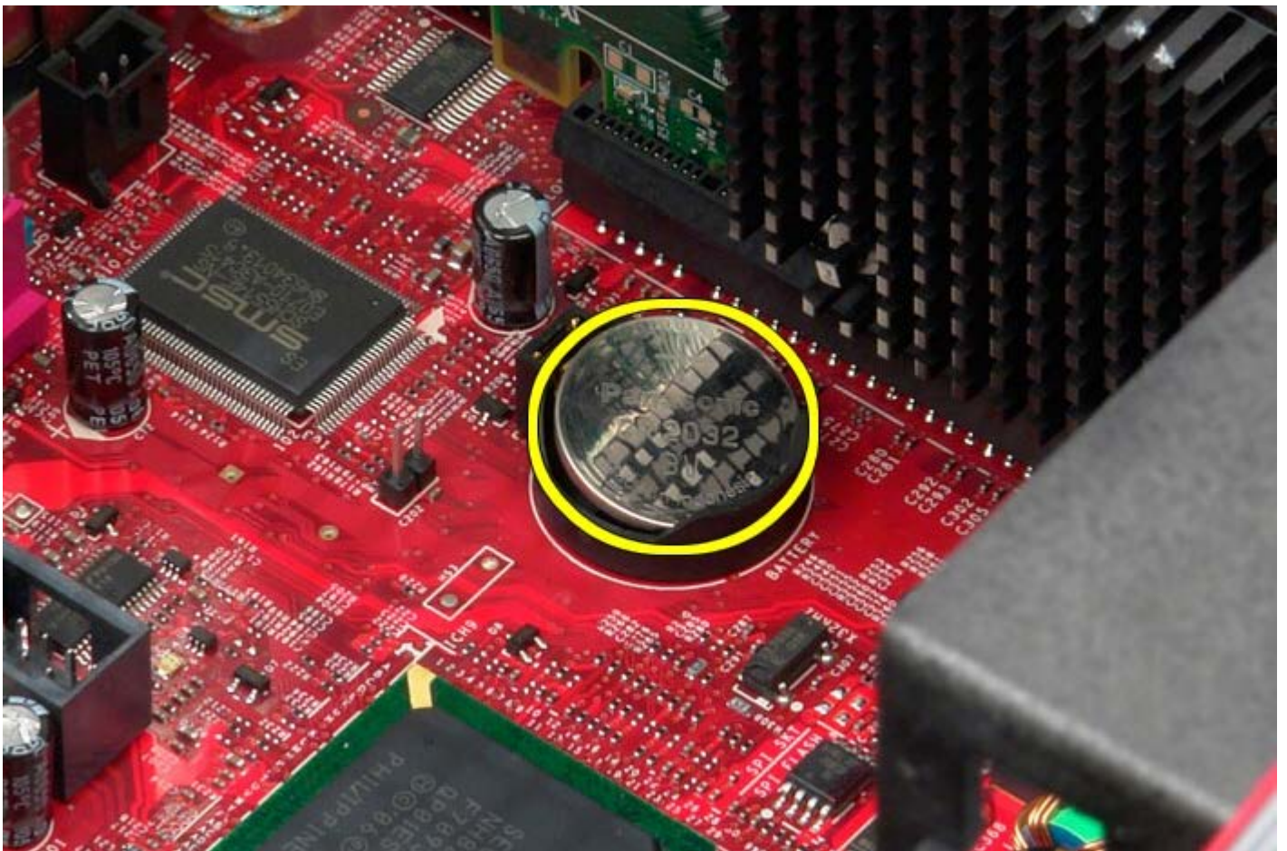
1 11 コイン型バッテリーをシステム基板から取り外します。
