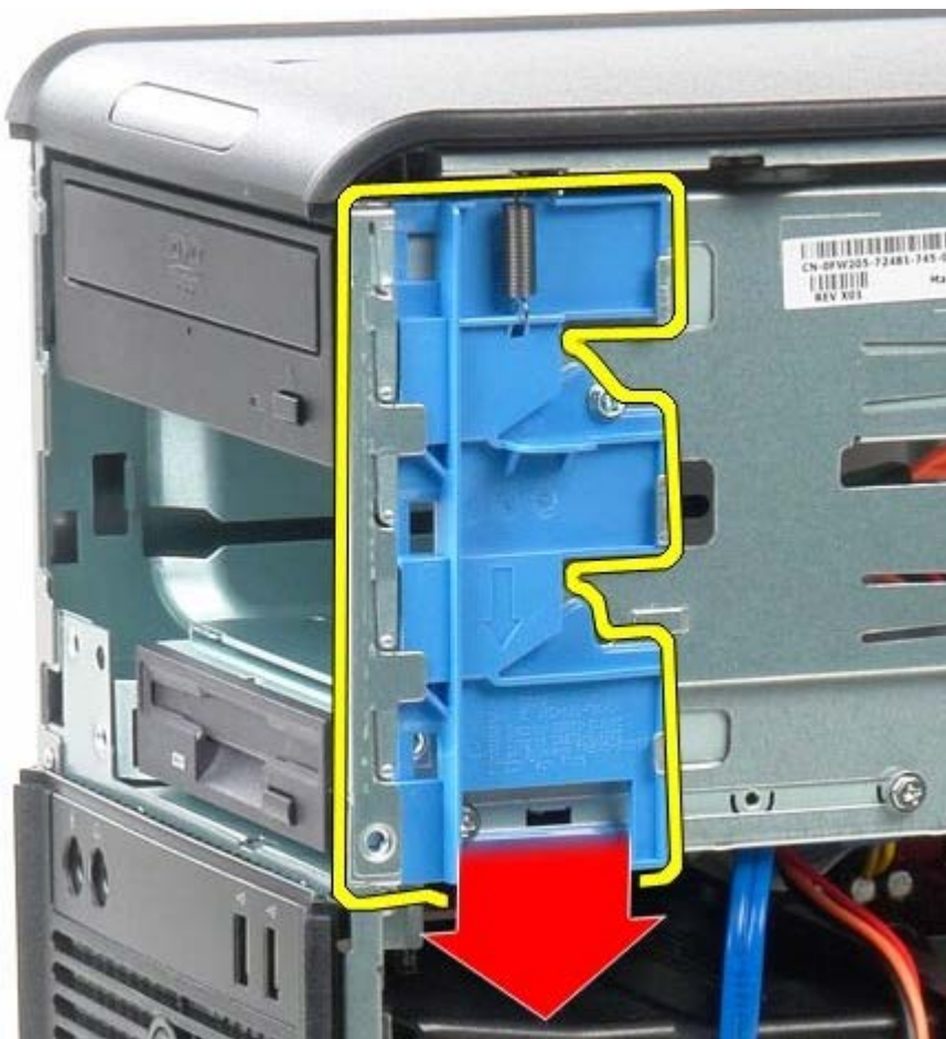
1 11 オプティカルドライブをシステムから引き出します。
