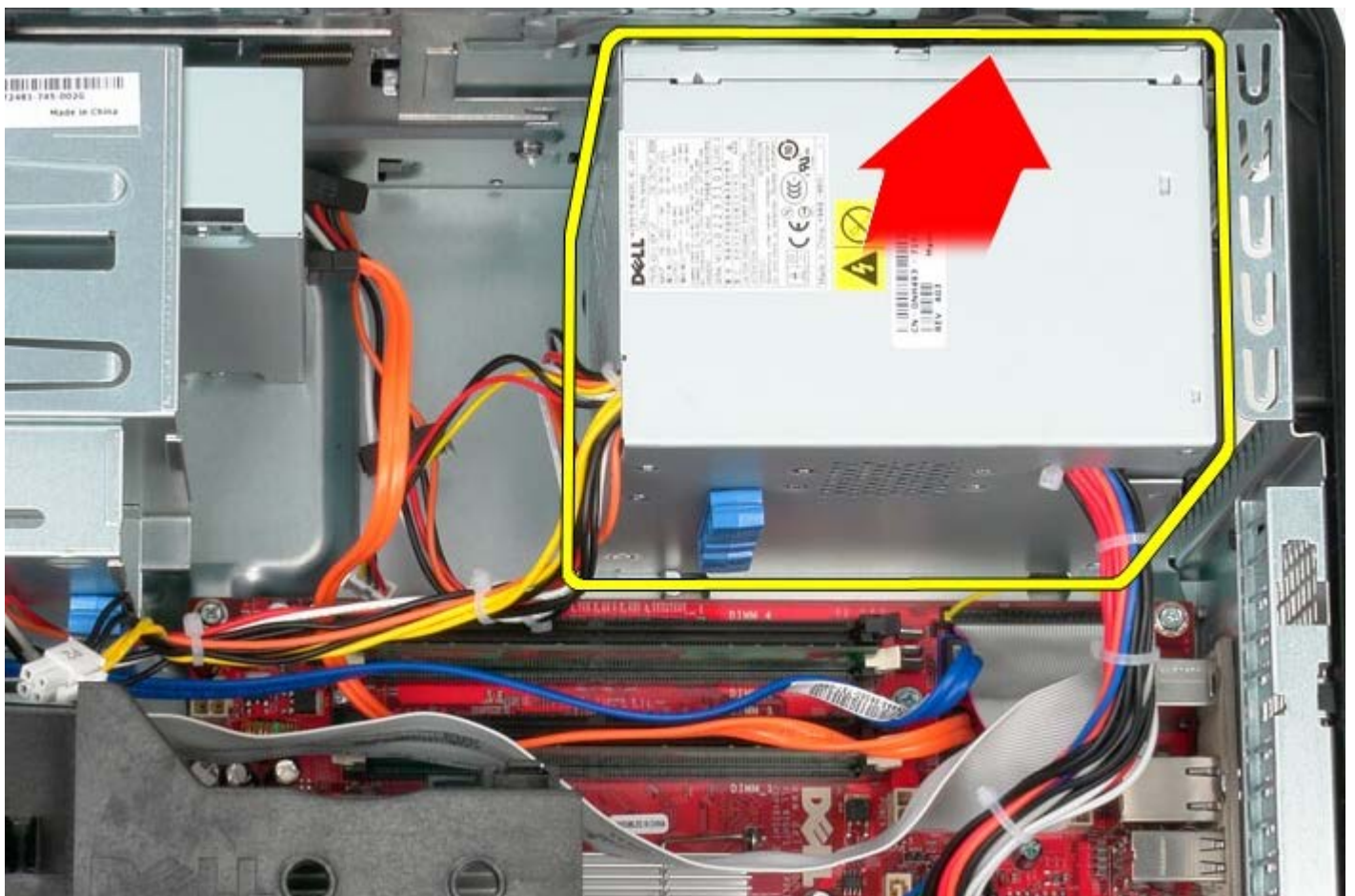
1 1 11 電源ユニットをコンピューターの前面に向かってスライドさせ、持ち上げながら、コンピューターから取り外します。
