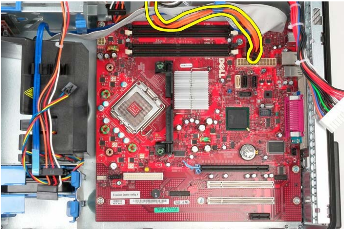
1 11 ハードドライブのデータケーブルをシステム基板から外します。
