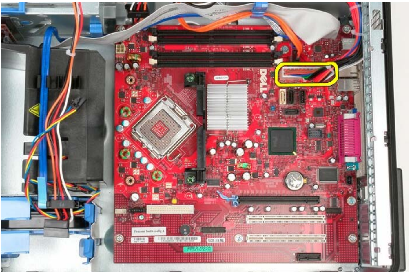
1 11 オプティカルドライブのデータケーブルをシステム基板から取り外します。
