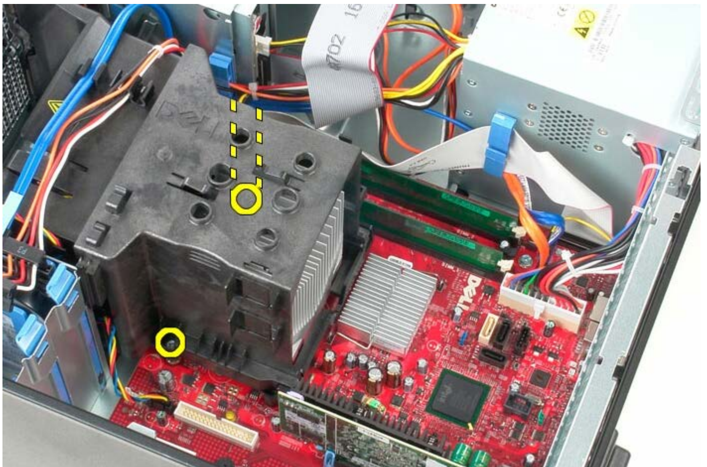
1 11 ヒートシンクをコンピューターの背面に向かって回します。
