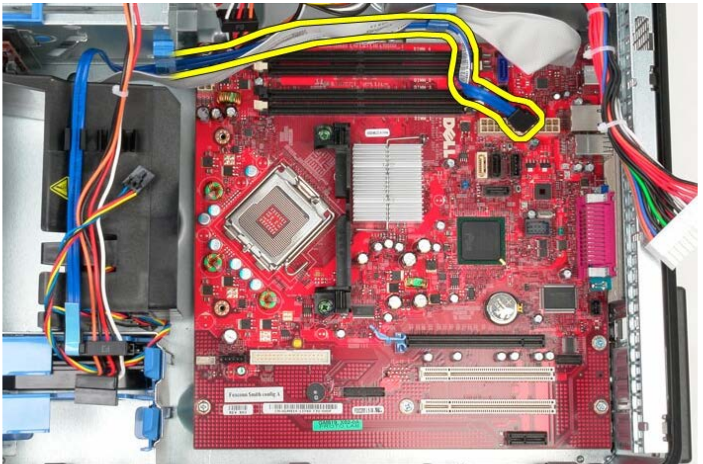
11 11 IO パネルのデータケーブルをシステム基板から外します。
