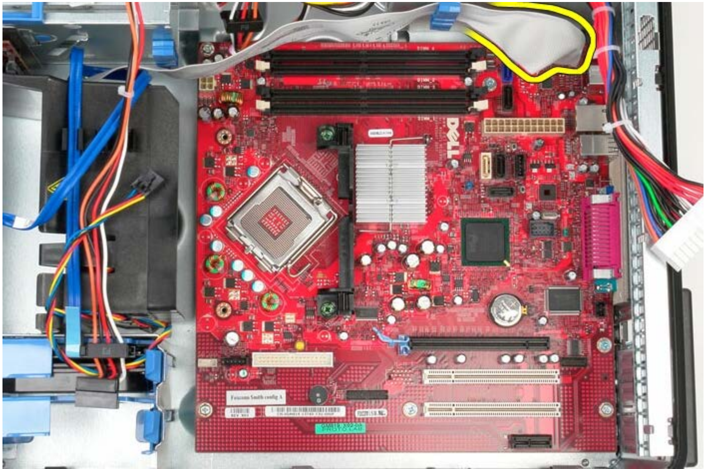
1 1 11 IO パネルケーブルを片付けておきます。
