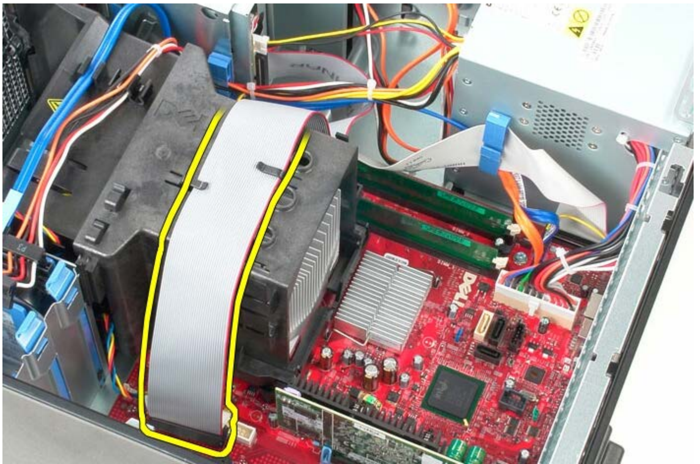
1 11 ヒートシンクをシステム基板に固定している 2 本の拘束ネジをゆるめます。
