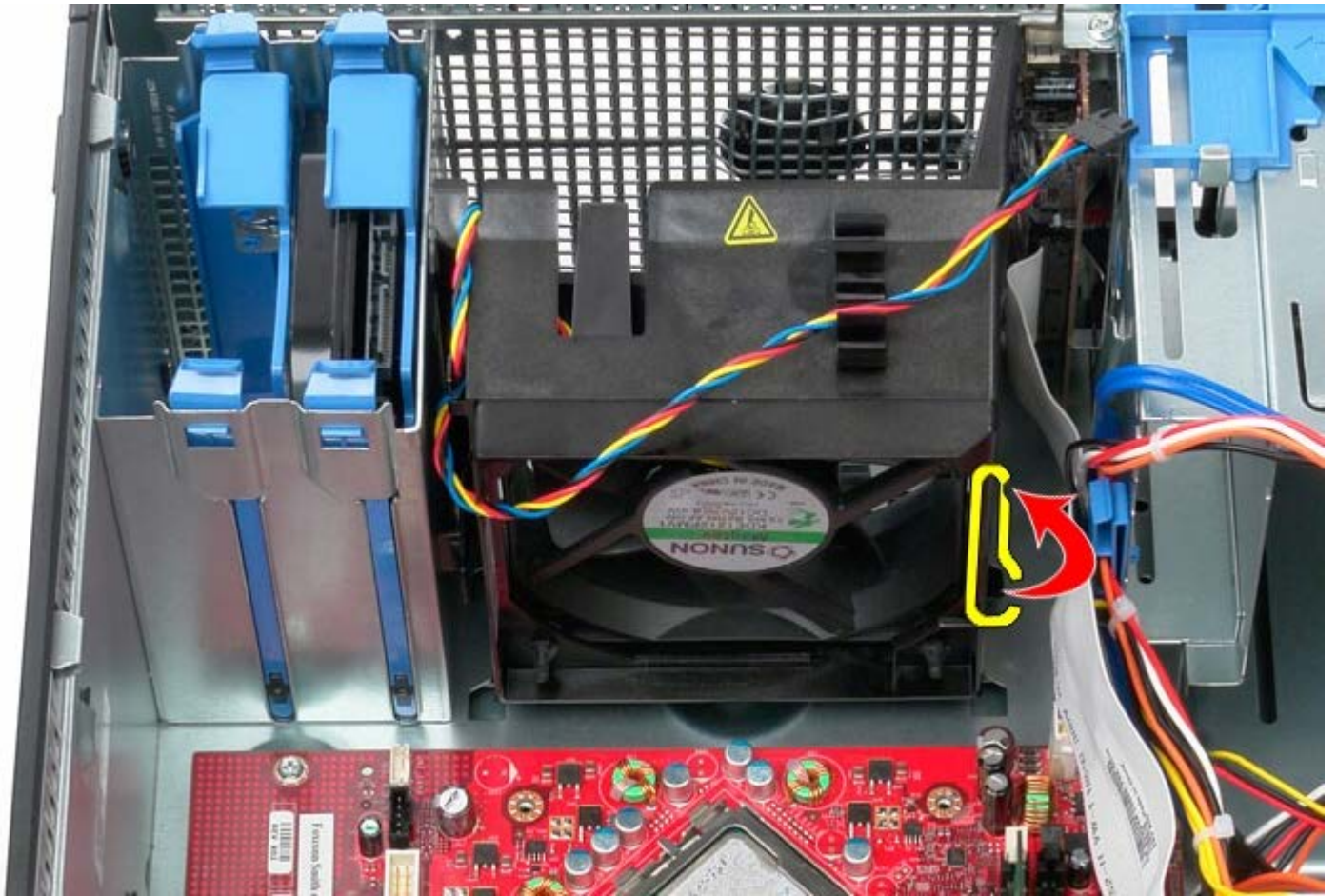
1 11 コンピューターの底面に最も近いプロセッサファン固定タブを押します。
