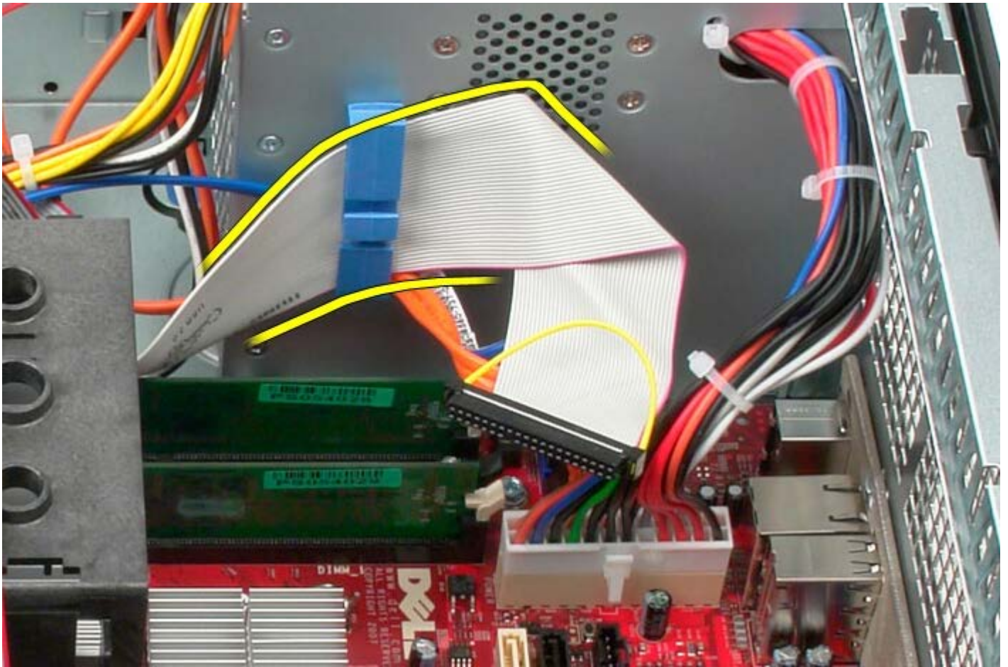
1 11 システムの前面に IO パネルを固定しているネジ 1 本を取り外します。
