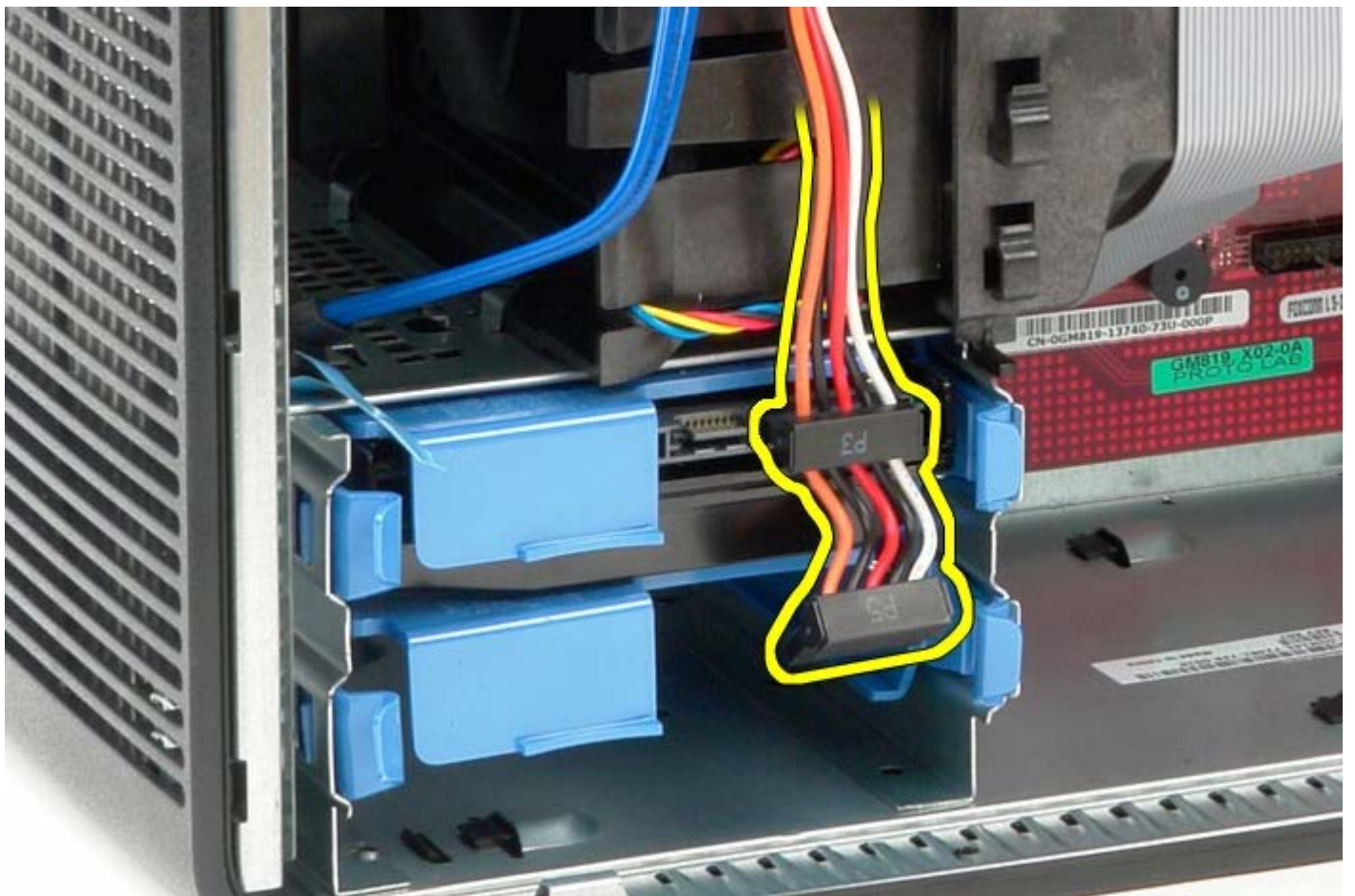
1 11 ハードドライブの両端にある青いリリースタブを押し入れます。
